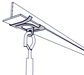
Clip en T-barre
